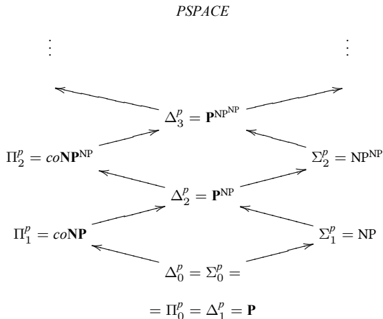
Σχήμα: Πολυωνυμική ιεραρχία
