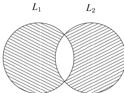
Σχήμα: Ισοδυναμία πεπερασμένων αυτομάτων
