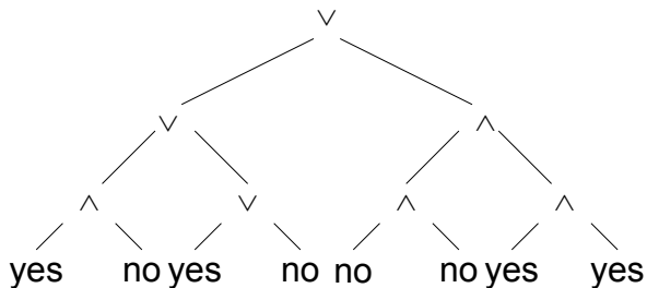
Σχήμα: Υπολογιστικό δένδρο με εναλλαγές
